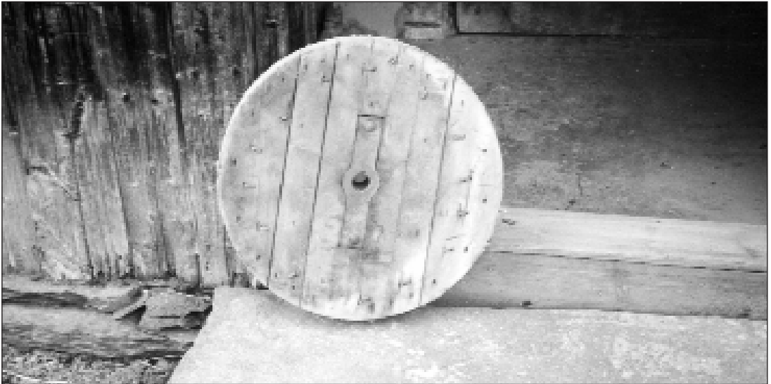
På Enge er det fortsatt en del igjen av jernhesten. Denne reimskiva av tre var festet til akslingen på jernhesten. Innenfor den, på akslingen, var det nok en reimskive som satt løst på akslingen som drivreima ble penset over på når vaieren skulle trekkes ut igjen.
