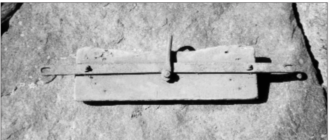
Når jernhesten ble brukt til lokjøring på Enge ble denne innretningen satt i skjekene på en høyvogn eller hjulslede. Det var da enkelt å skifte ut fra jernhesten til en vanlig hest.
